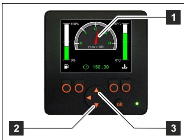
Afb. 92: display met functietoetsen - machinestart dieselmotor
