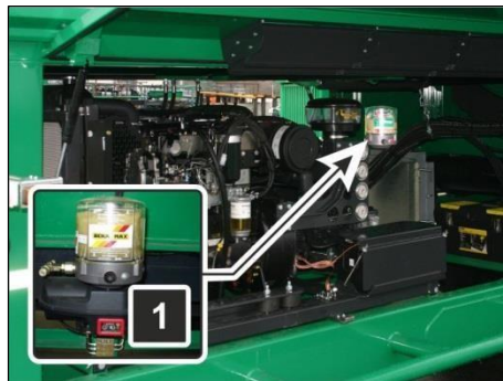
Afb. 20: centrale smeereenheid
