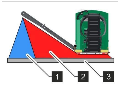
Afb. 69: vrije ruimte onder de machine - achter
