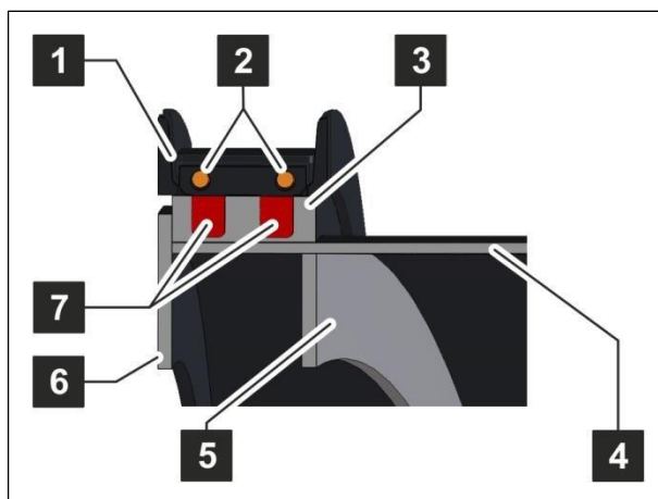
Afb. 106: zeeftrommel SM620 - detail spaanelement
