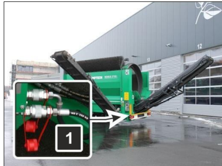
Afb. 14: extra hydraulische aansluiting - snelkoppelingen
