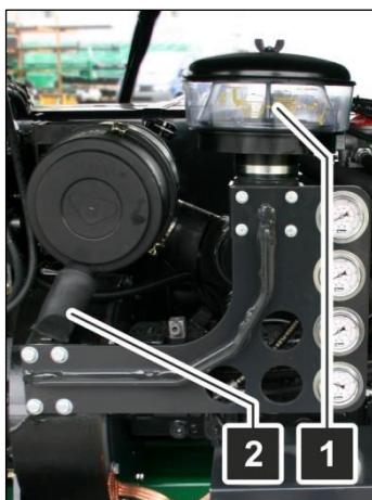
Afb. 79: motor - luchtfilter- voorafscheider XE "Luchtfilter"
