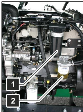
Afb. 77: brandstoffilter en waternuwaarscheider XE "Waternuwaarscheider"
