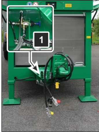
Afb. 67: losventiel persluchtstelsysteem
