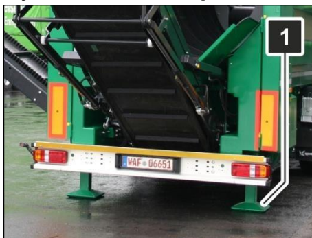
Afb. 33: extra achterstempel
