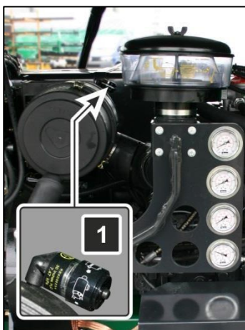
Afb. 78: luchtfilter - vervuilingsindicatie XE "Luchtfilter"
