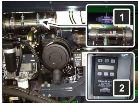
Afb. 36: motor - roetfilter
