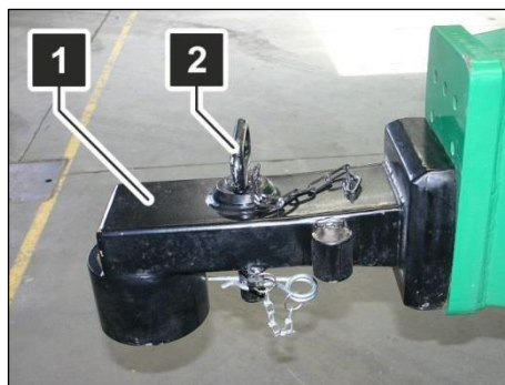
Afb. 18: opzetschoen
