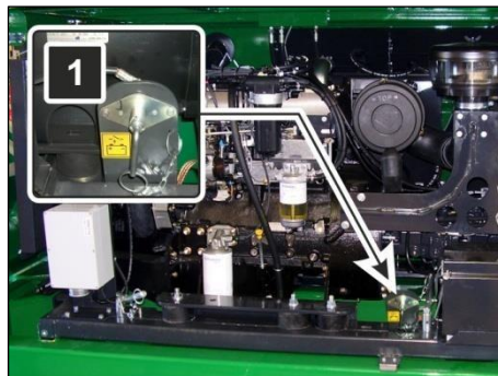
Afb. 37: accuscheidingsschakelaar
