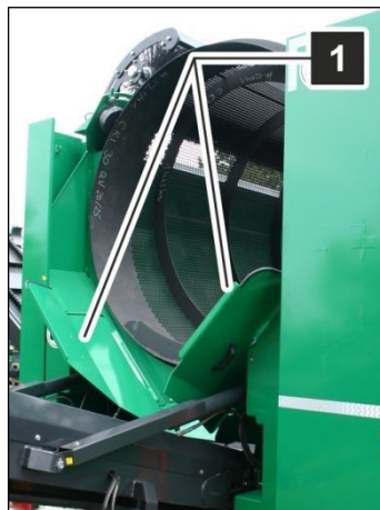
Afb. 51: zwenkbare uitloopgoot
