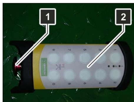
Afb. 22: afstandsbediening
