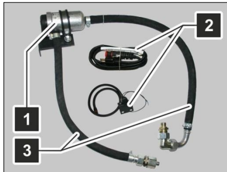
Afb. 25: motorvoorverwarming
