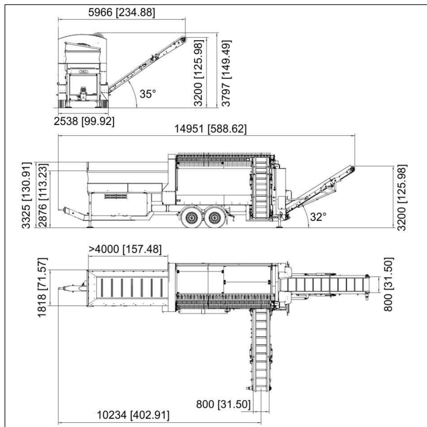
Afb. 5: afmetingen bedrijfsstand
