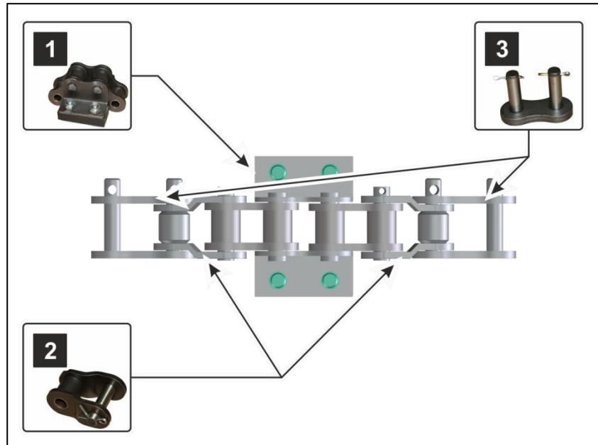
Afb. 109: zeftrommel SM620 - verlengen aandrijfketting
