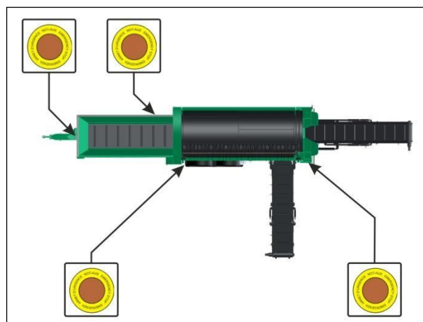
Afb. 2: veiligheidsinrichtingen
