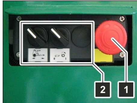
Afb. 61: bedieningspaneel 4 - bedieningselementen
