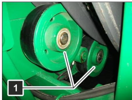
Afb. 32: tandendraagwielen
