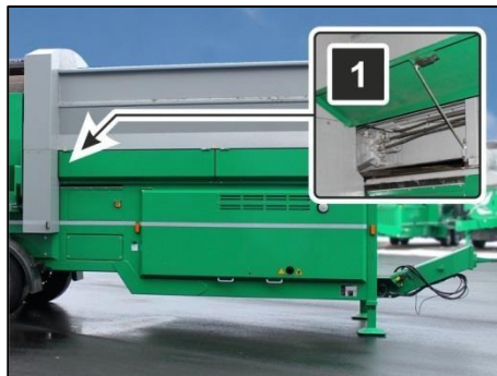
Afb. 71: motorreductor bunkerband
